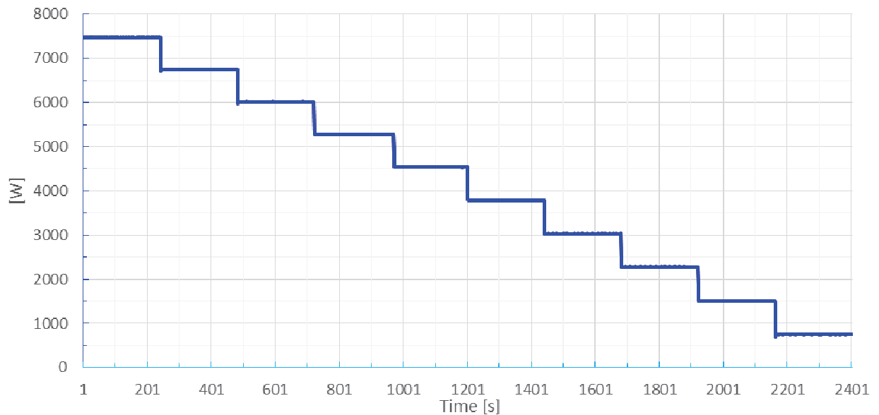
Gráfico limitação da potência activa em coincidência com comando remoto Graph active power limitation in adjusted with remote control
