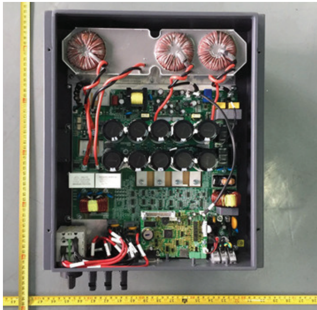
Figura 3. Visão interna-1 Figure 3. Internal view-1
